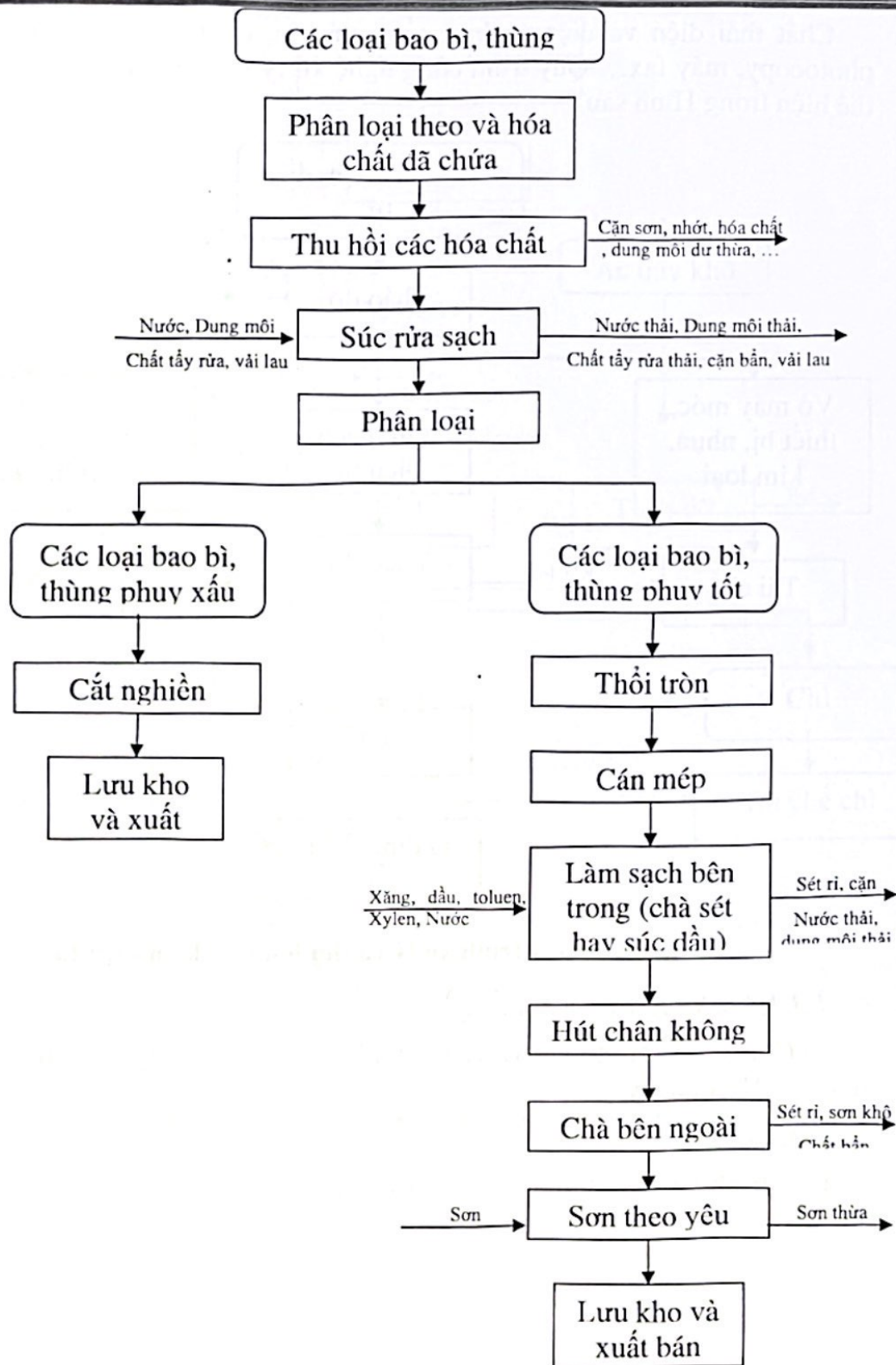
Hình 6: Quy trình súc rửa và phục hồi bao bì, thùng phuy
