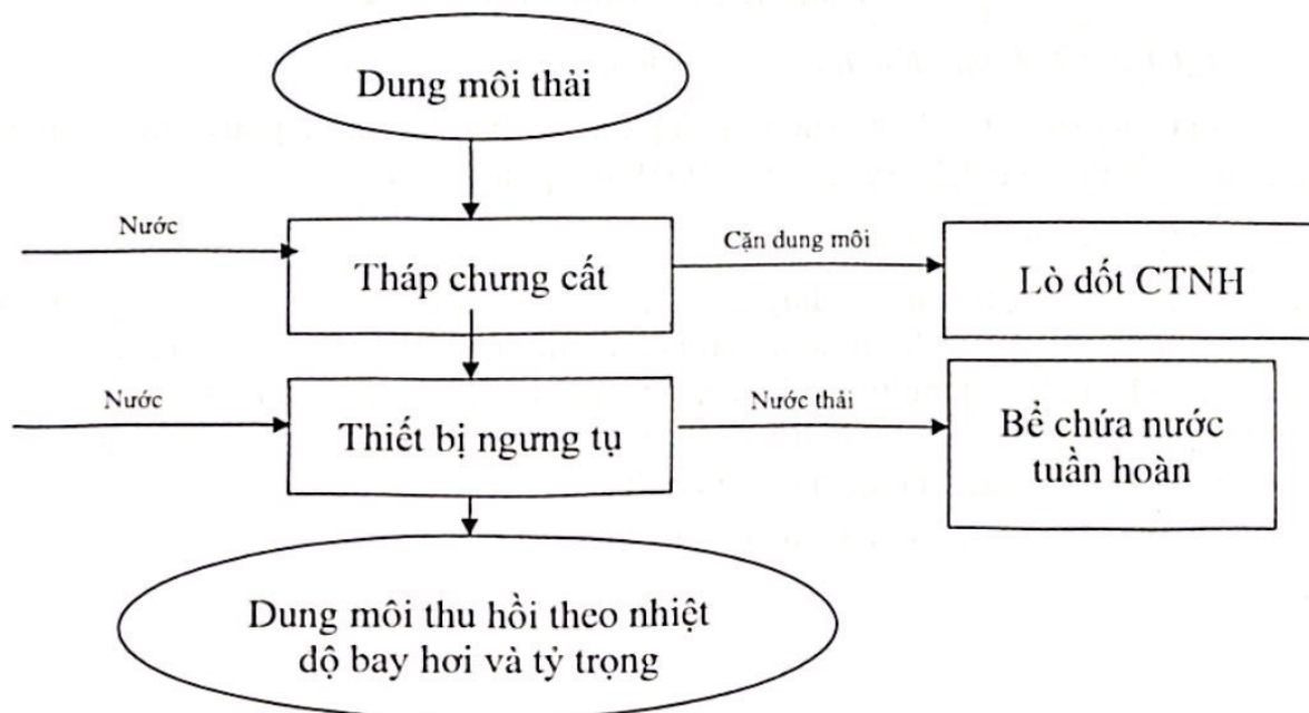
Hình 3. Quy trình tái chế dung môi
