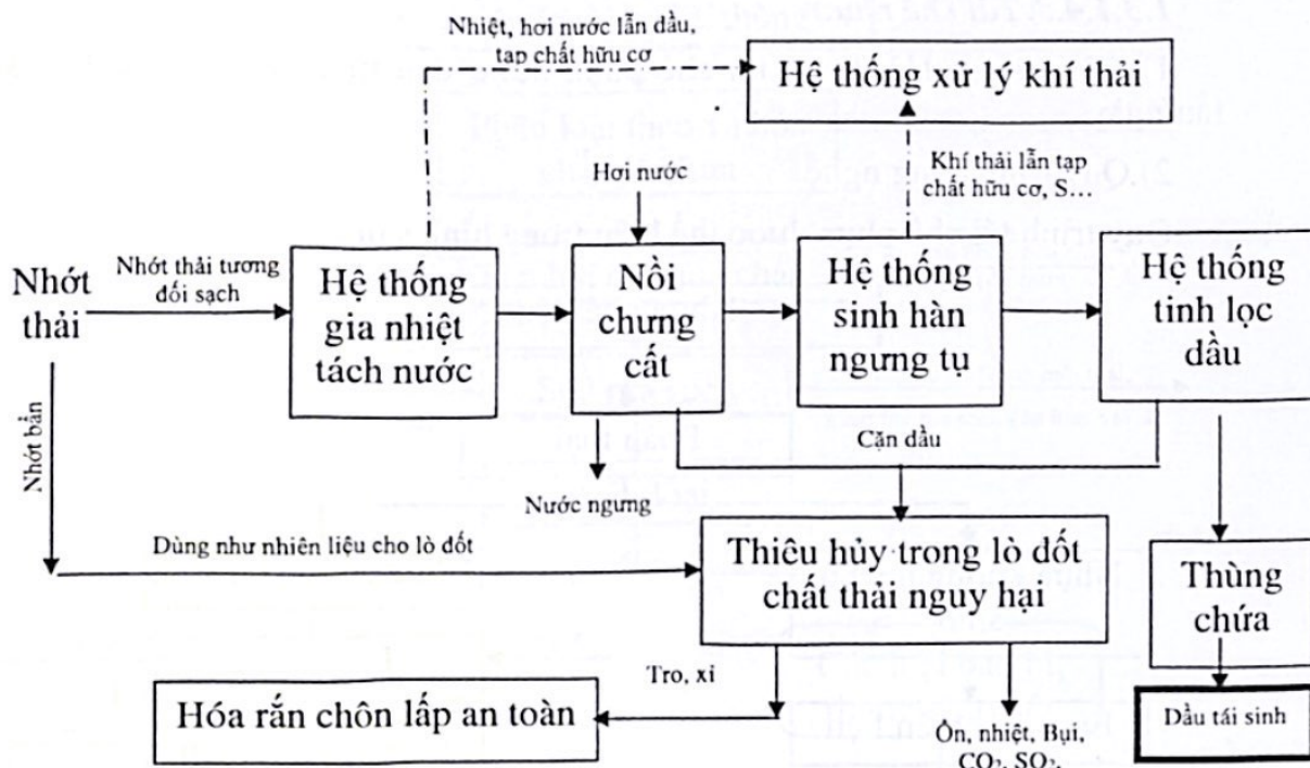
Hình 2. Quy trình tái chế dầu nhớt thải
