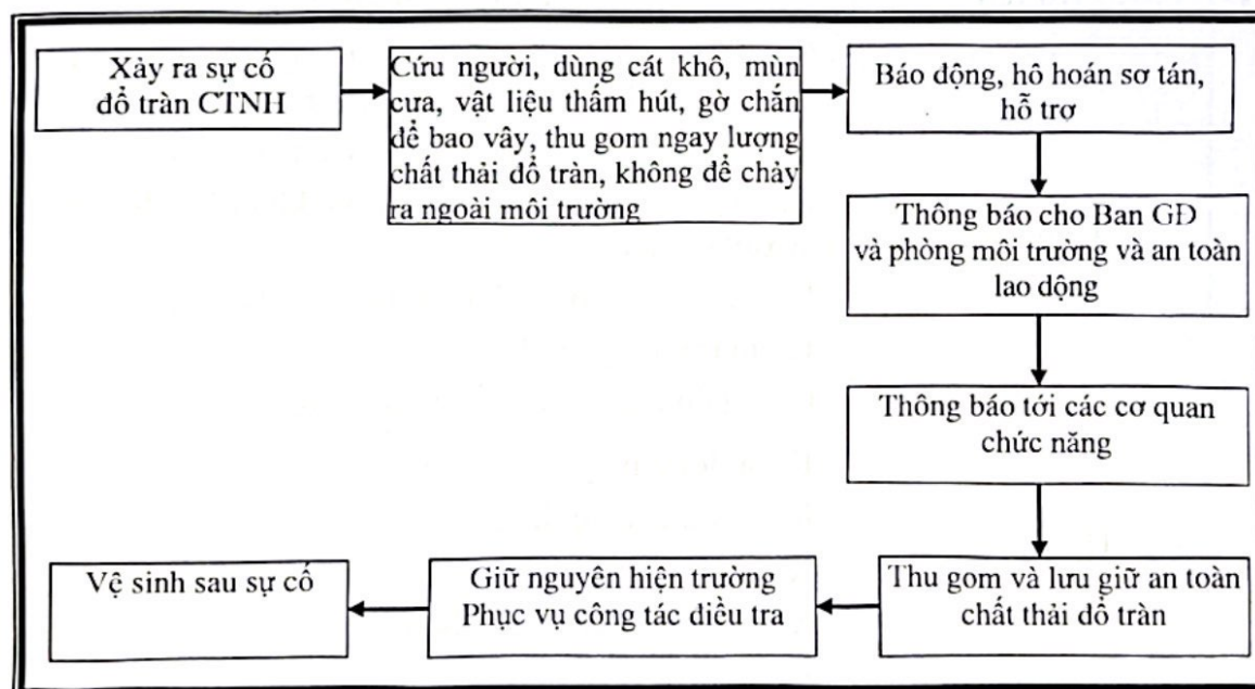
Hình 25: Sơ đồ hướng dẫn ứng phó khẩn cấp trong trường hợp xảy ra tai nạn lao động
