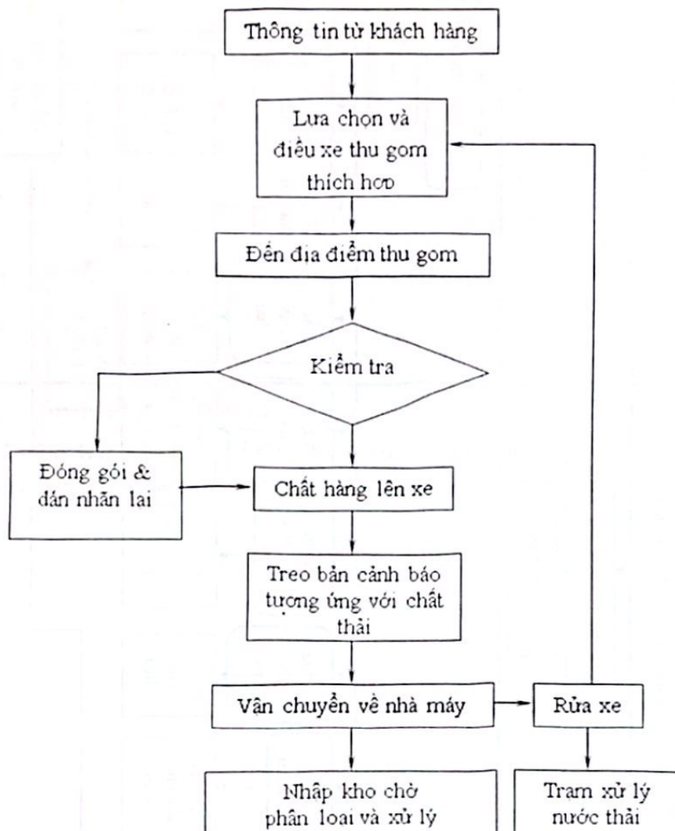
Hình 1. Sơ đồ quy trình thu gom và vận chuyển chất thải
