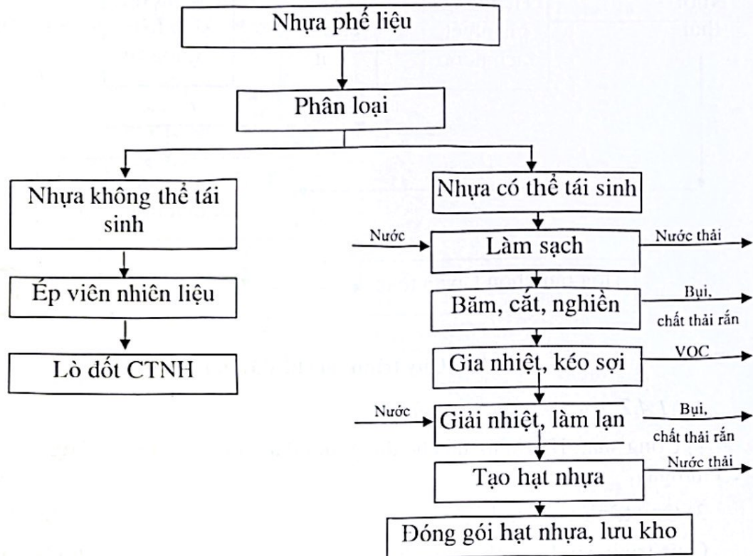
Hình 1. Quy trình tái chế nhựa
