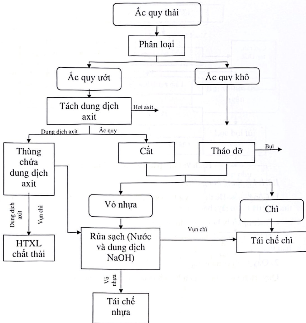
Hình 8: Quy trình xử lý và thu hồi ắc quy
