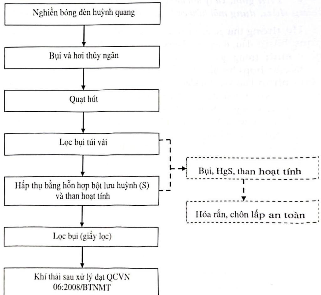
Hình 21: Quy trình xử lý bụi và hơi thủy ngân từ dây chuyền xử lý bóng đèn
